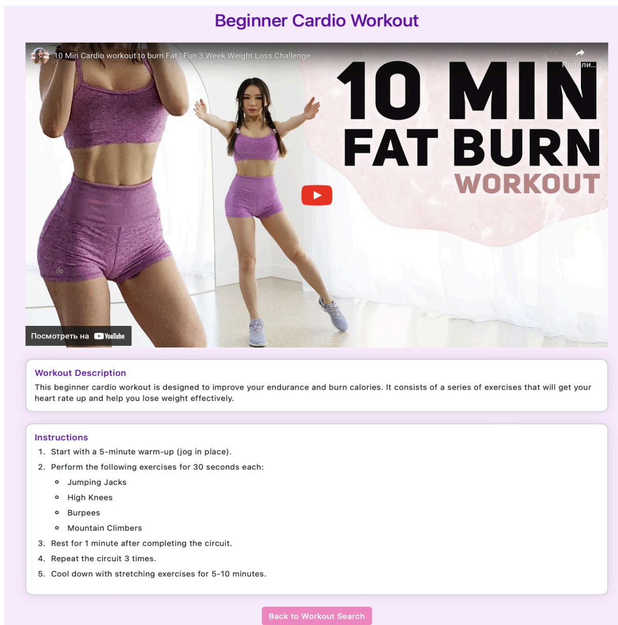
Рисунок 6 - Страница тренировки
